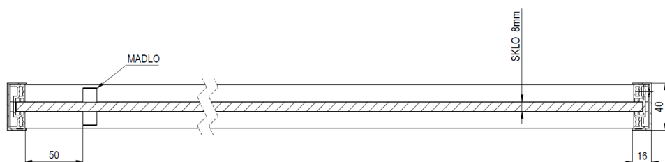
Řez vodorovný
